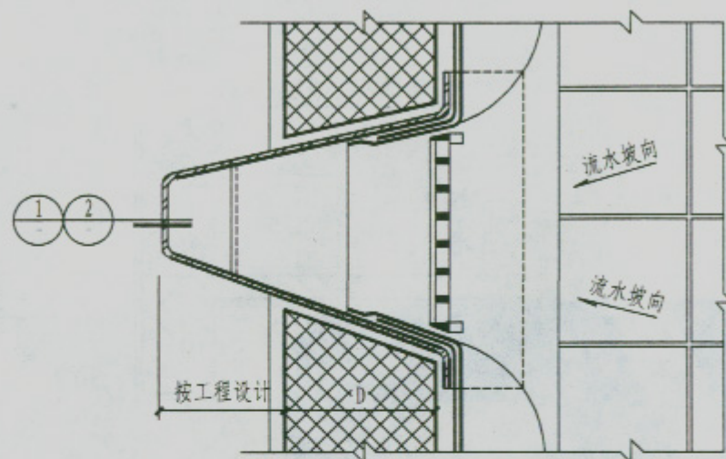
平面
