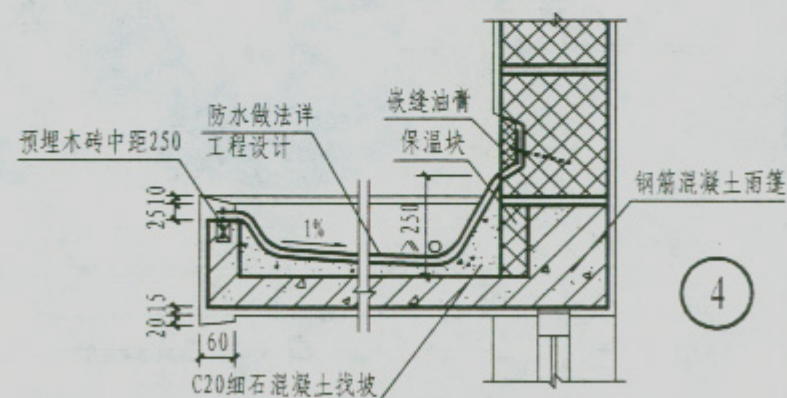
女儿墙及雨篷详图(一)
