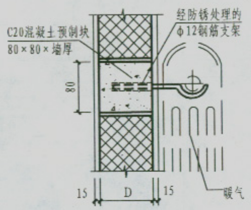
暖气片与墙体连接
