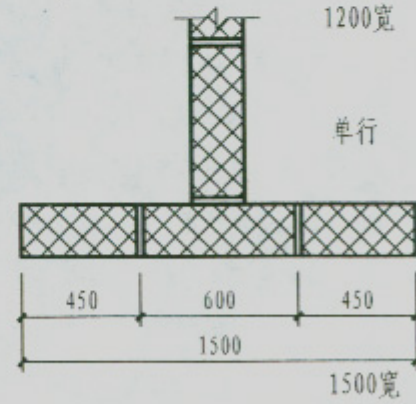
“T”型墙
