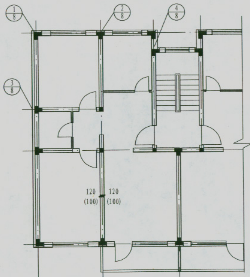
内砖外砌平面图
