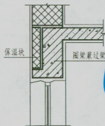
④ 外墙窗口
