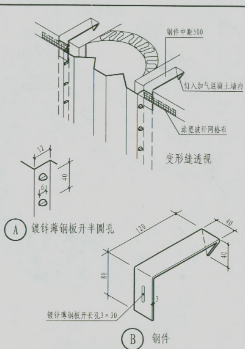
变形缝详图
