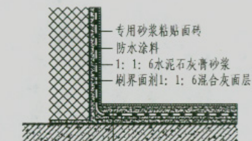
楼面做法
