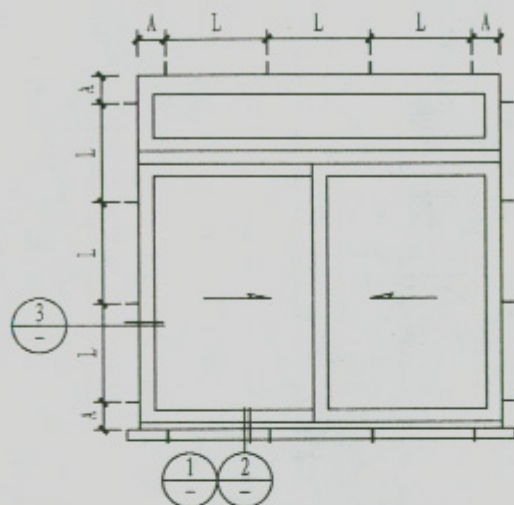
钢连接件位置立面图
