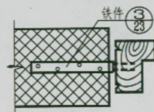
④ 先立框后砌墙门窗固定法
