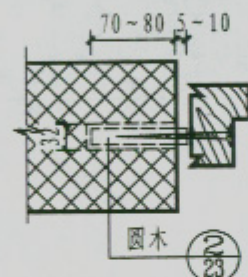
② 胶粘圆木安装法
