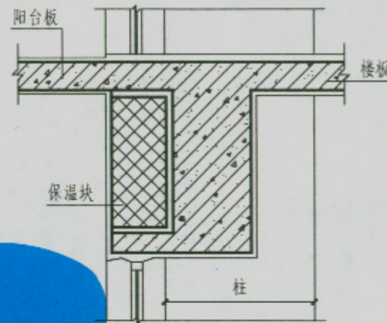
③ 阳台部位 (框架)
