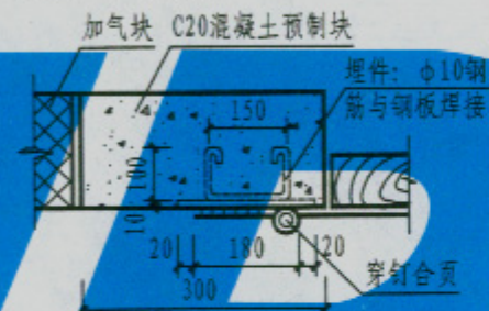
⑤ 重型门固定法 (适用于库房大门)
