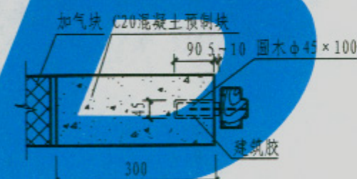
⑥ 重型门固定法 (适用于内门)
