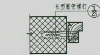
① 塑料胀管螺钉安装法
