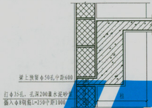
② 外墙 (框架)
