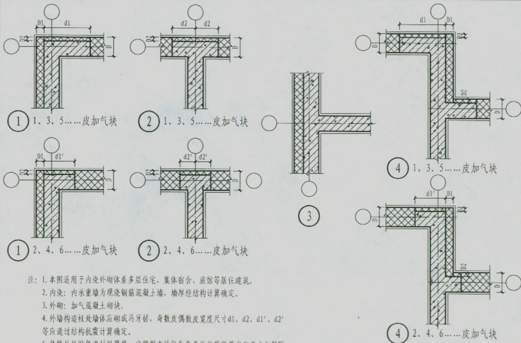
内浇外砌外墙构造详图
