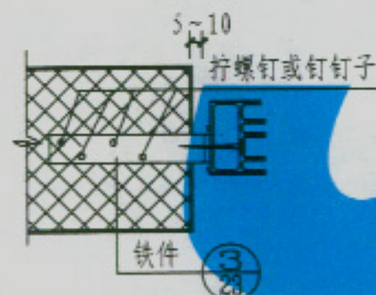
③ 铝合金及塑钢门窗安装法
