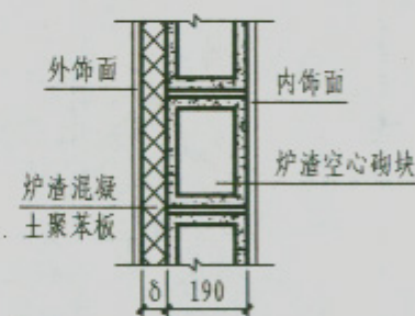
⑦ 潮湿房间外墙做法
