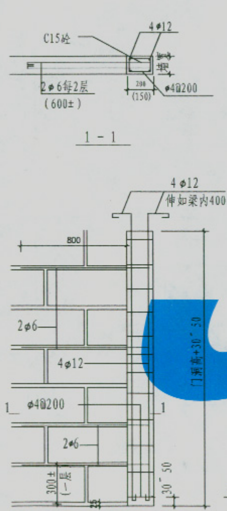
① 钢筋混凝土门框 (非承重墙)
