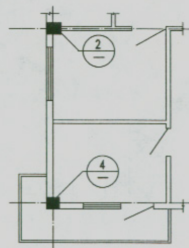
平面示例 (墙在柱间)
